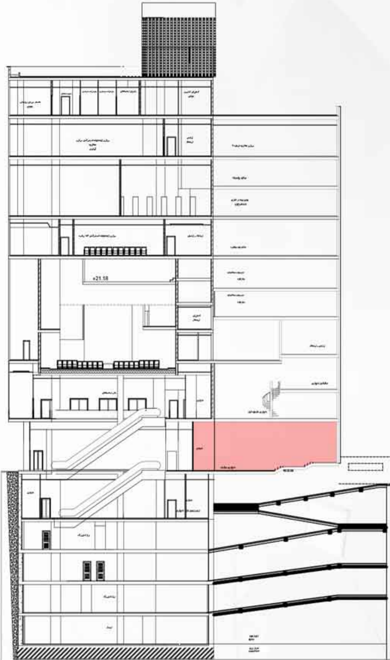
برش غربی
